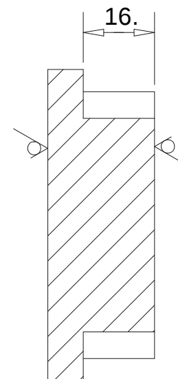
Leikkaus A-A
